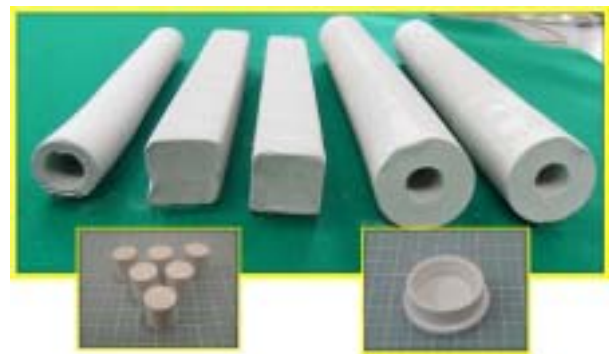
図5 押し出し成型品
